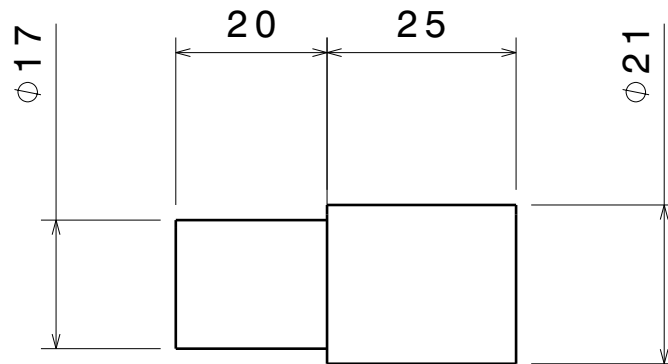
Vue de face Echelle : 1:1
