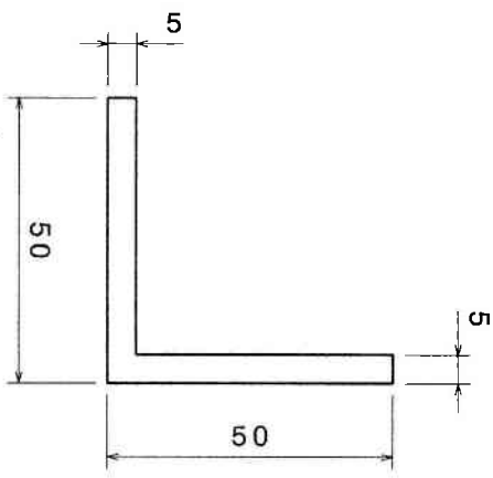
Détail B Echelle : 1:1
