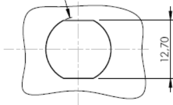
Détail C (2:1)
