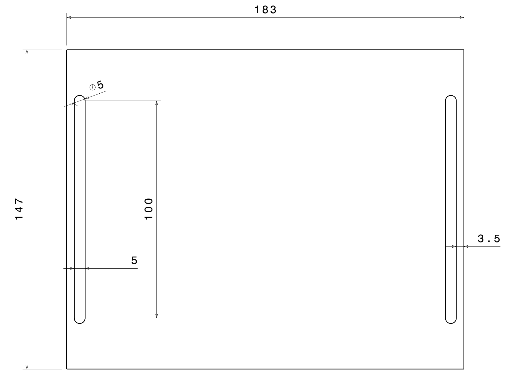
Vue de derrière Echelle : 1:1
