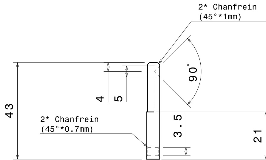
Vue de dessous Echelle : 1:1
