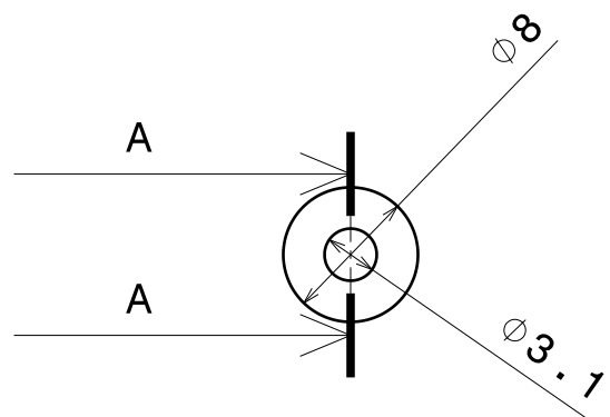
Vue de face Echelle : 2:1
