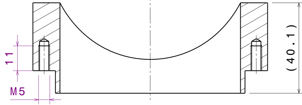
Coupe A-A Echelle : 1:1
