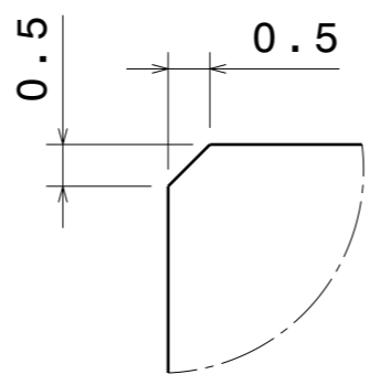
Détail B Echelle : 10:1
