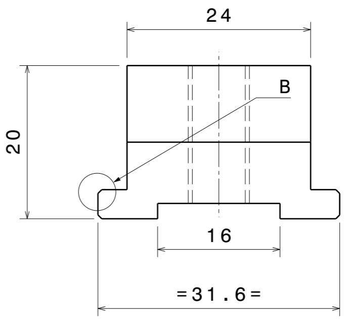
Vue de gauche Echelle : 2:1
