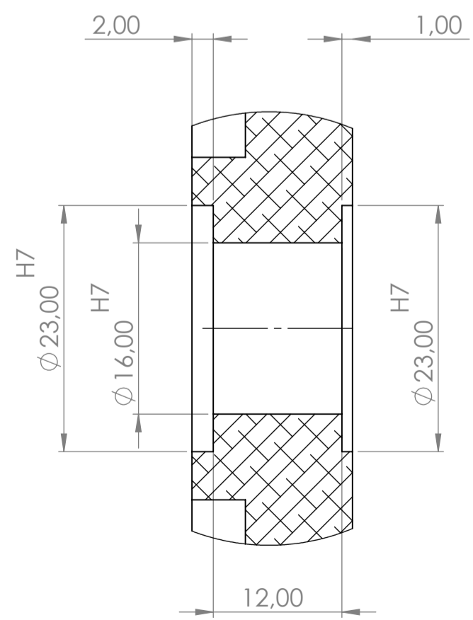
DÉTAIL B ECHELLE 2 : 1
