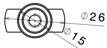
Vue de droite Echelle : 1:1
