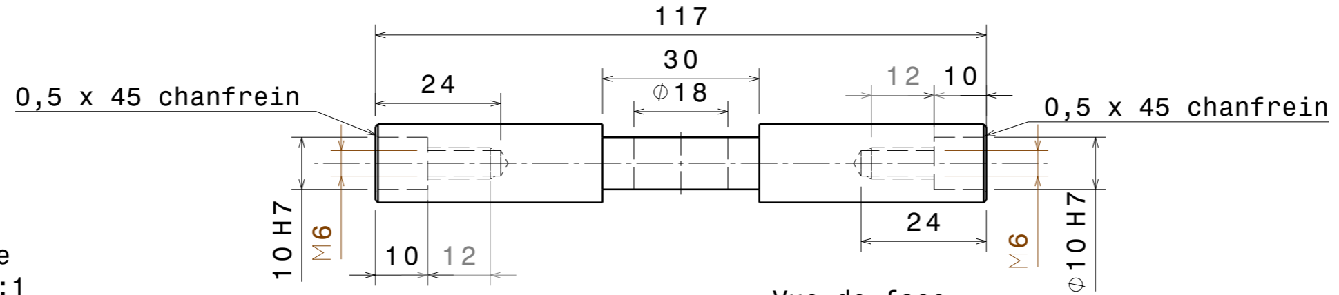
Vue de face Echelle : 1:1
