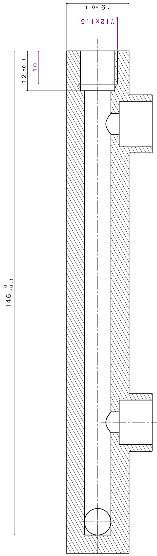
B-B Echelle : 5:1
