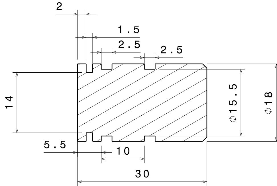
Coupe A-A Echelle : 2:1
