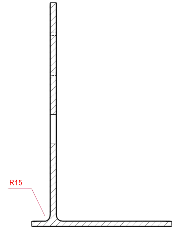
Coupe A-A
