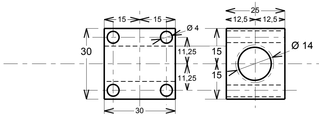
ecrou trapezoidal de 14x3 a droite
