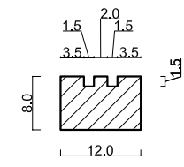
Coupe CC pièce_3
