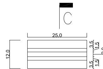
Plan pièce_3
