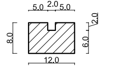
Coupe BB pièce_2
