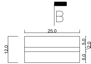
Plan pièce_2
