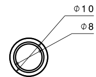
Left view Scale: 2:1
