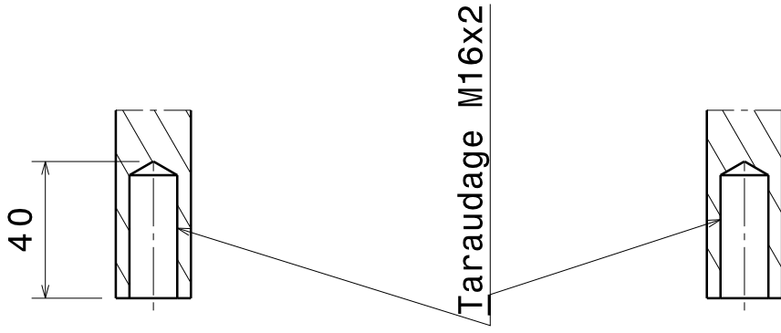
Coupe A-A Echelle : 1:2
