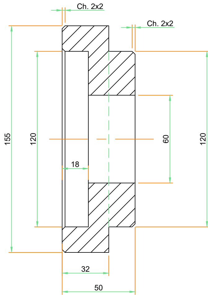
Coupe A-A
