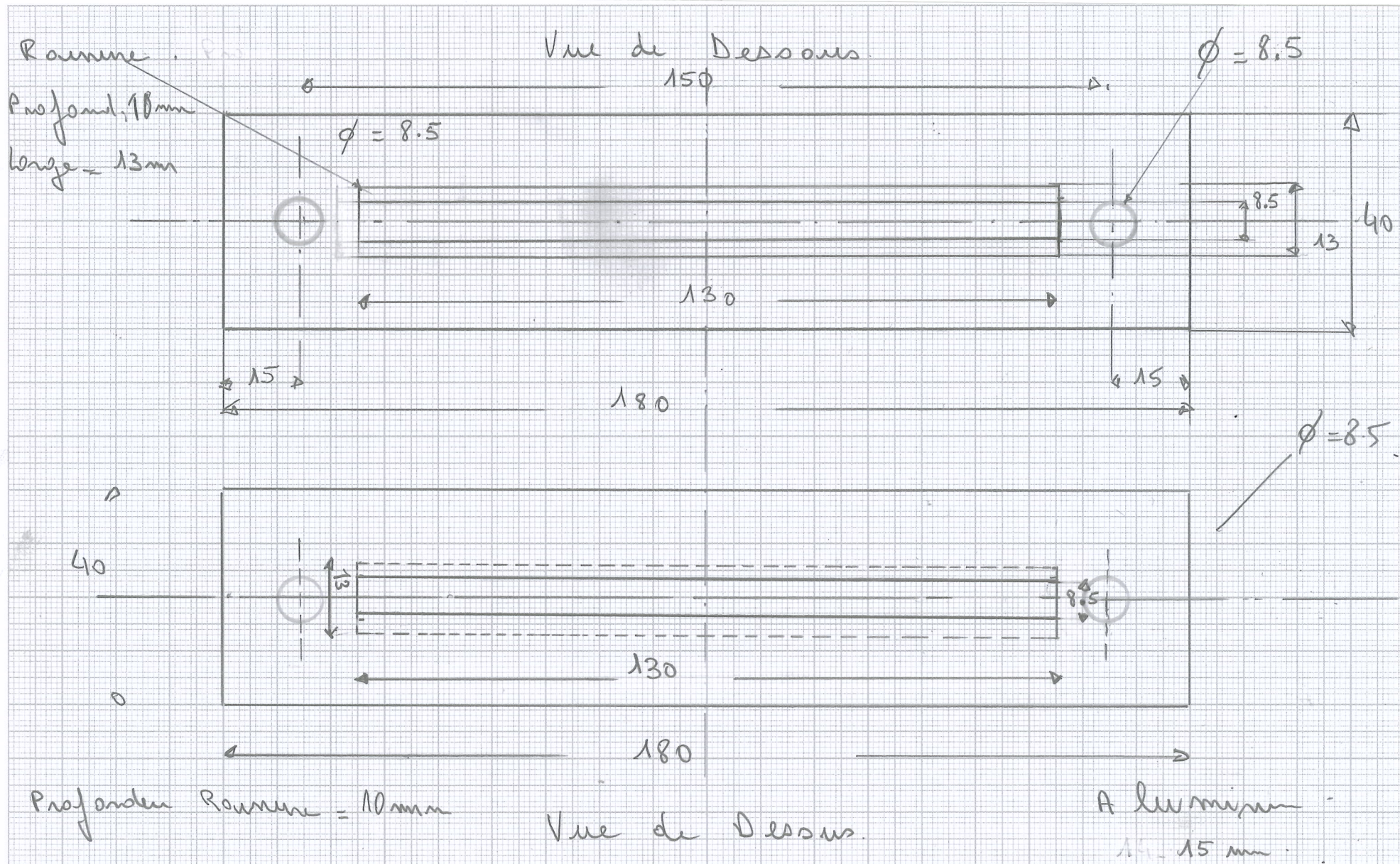
BRIDE AJUSTEMENT VERIN PORTAIL
