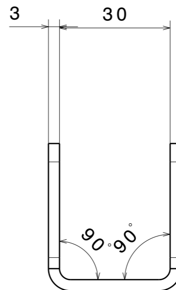
Vue de gauche Echelle : 1:1
