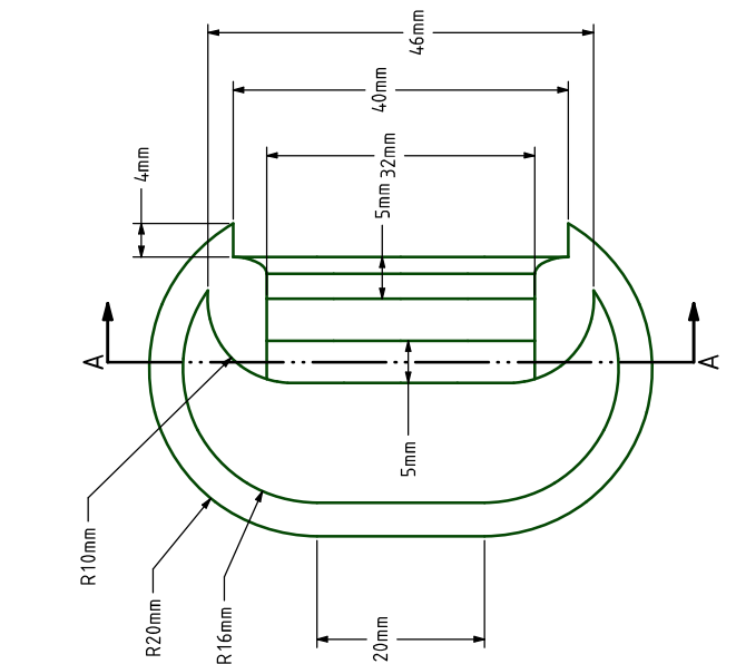
M3 débouchant avec filetage Ø17 prof: 3
