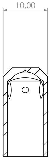
COUPE A-A
