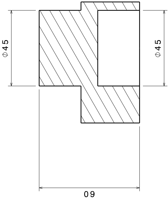
Coupe A-A
