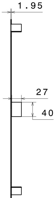
Vue de face Echelle : 1:5
