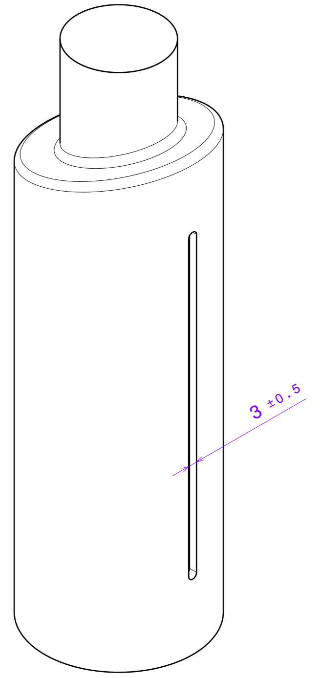
Vue isométrique Echelle : 1:1
