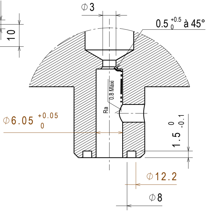
Détail A
