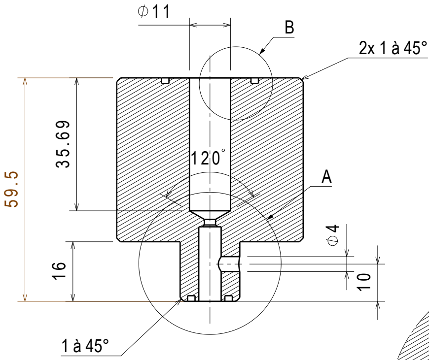
Coupe A-A
