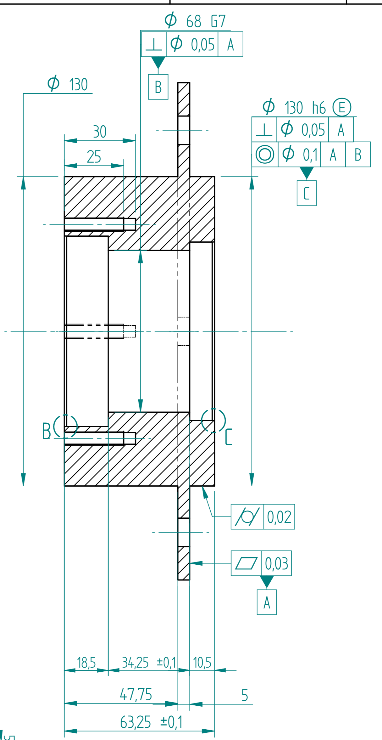
SECTION A-A
