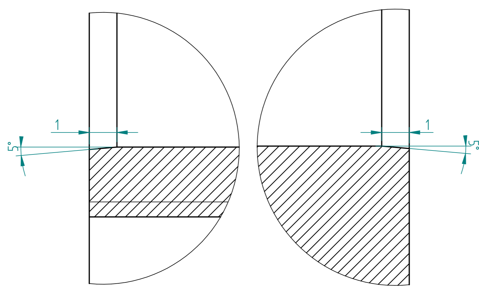
DETAIL B Echelle 12:1 DETAIL C Echelle 12:1
