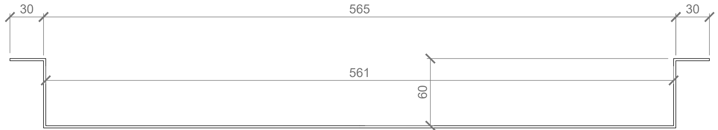
COUPE AA
