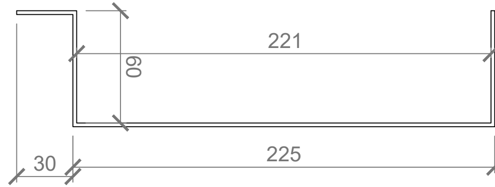
COUPE BB
