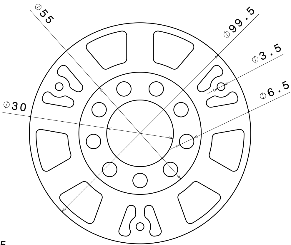
Vue d'en Bas Echelle : 1:1
