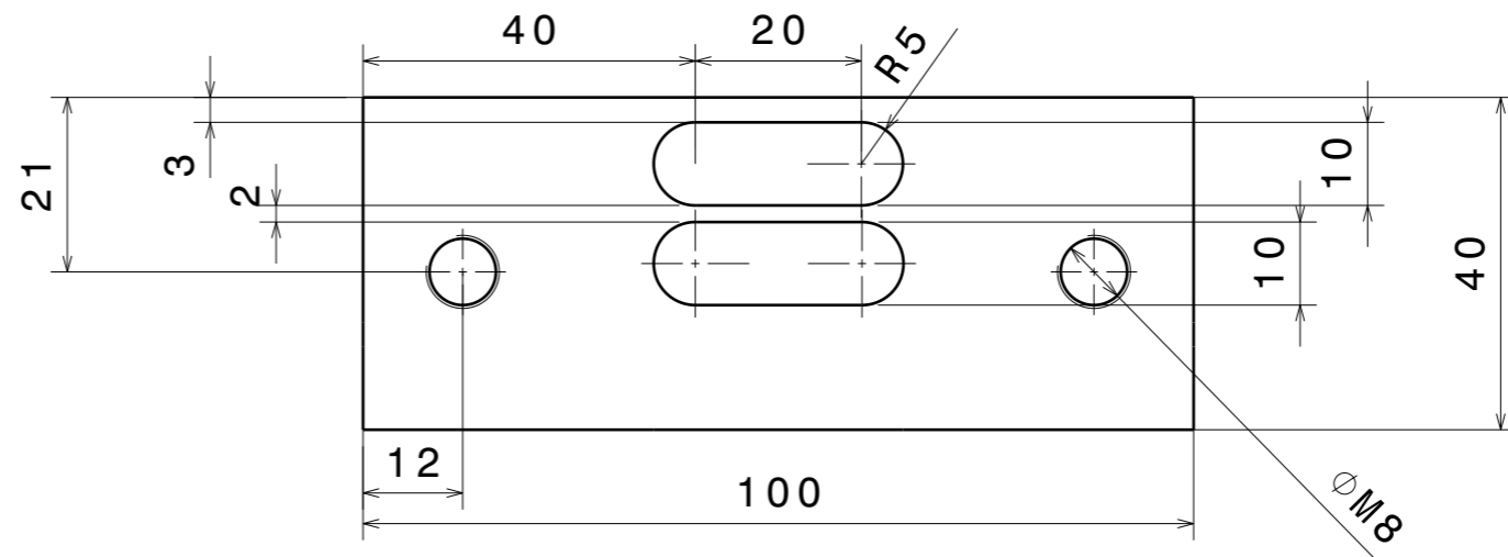
Vue de dessous Echelle : 1:1
