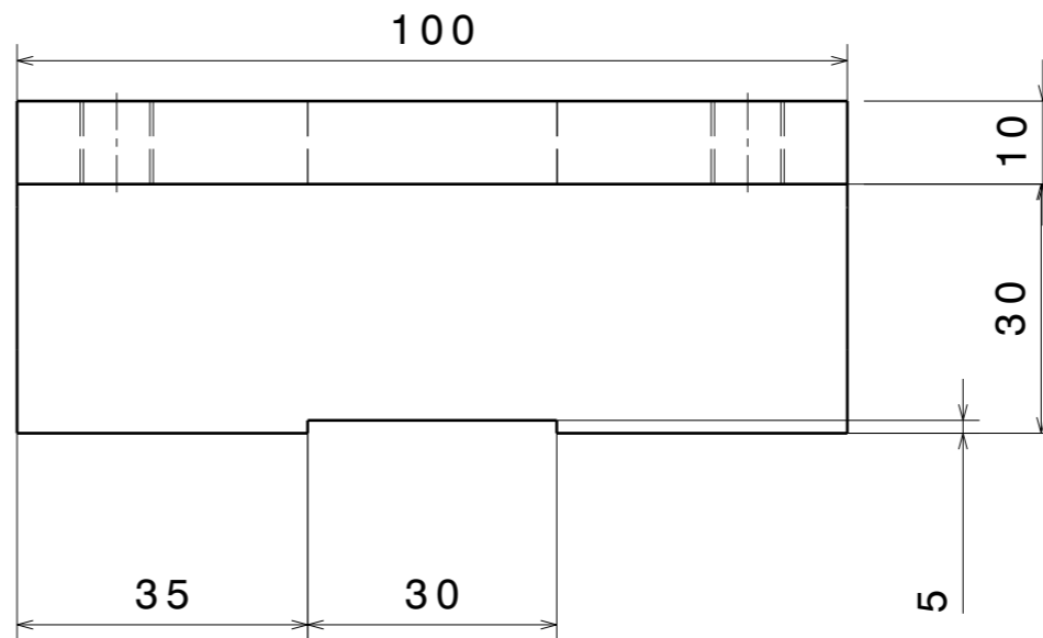
Vue de face Echelle : 1:1
