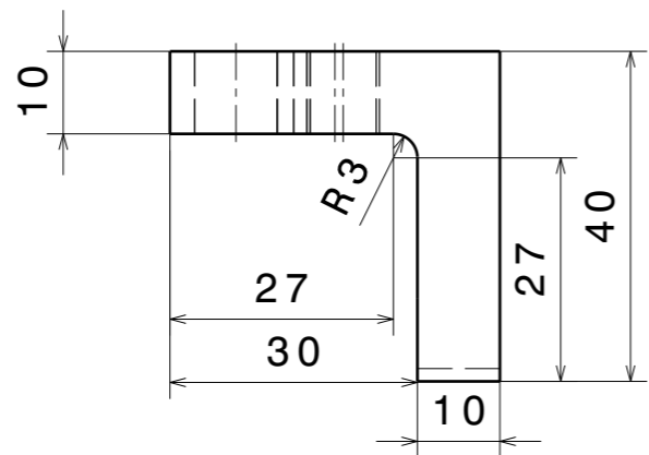
Vue de droite Echelle : 1:1
