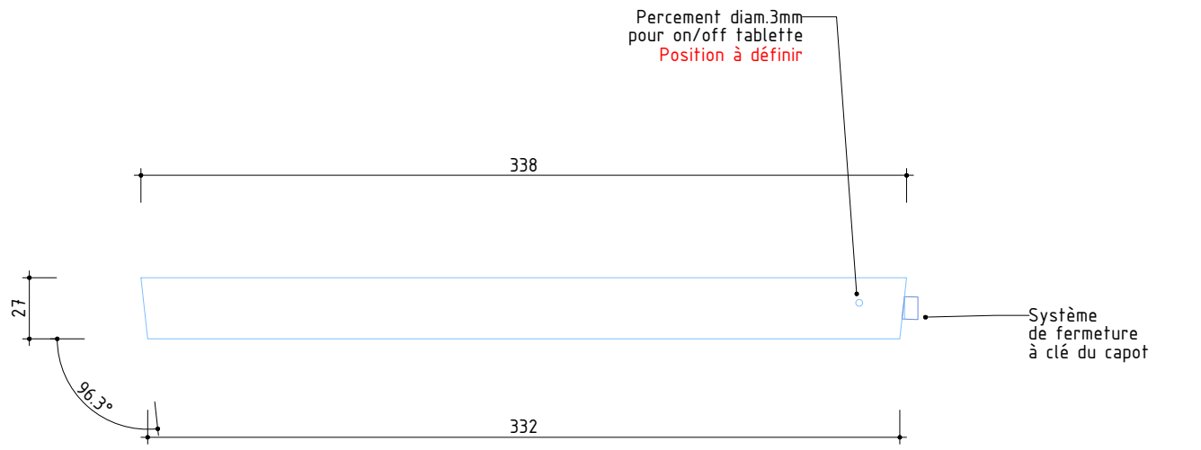
VUE FACE BOITIER
