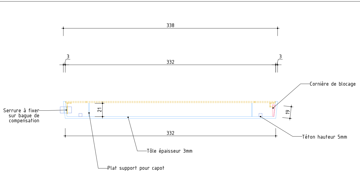
COUPE BOITIER
