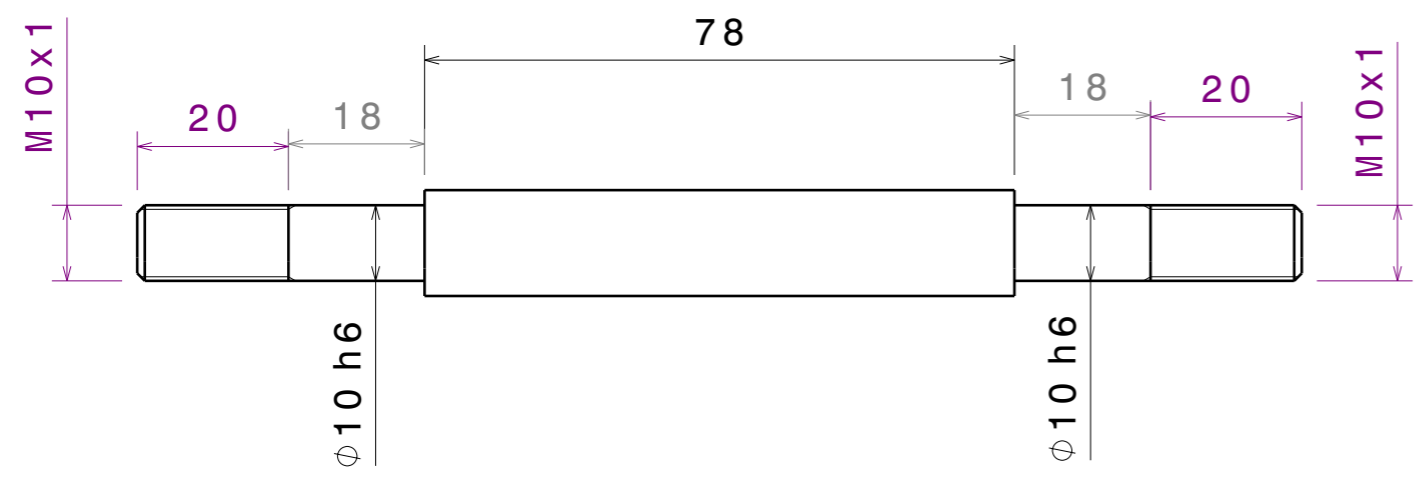
Front view Scale: 1:1
