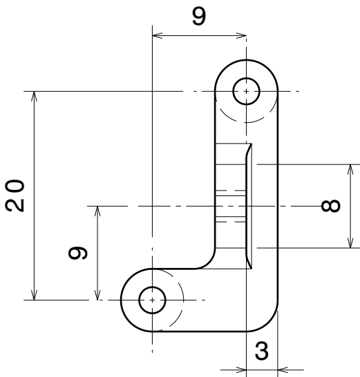
Top view Scale: 2:1
