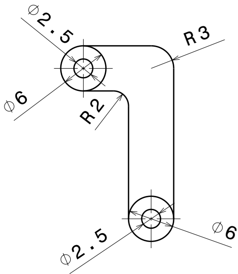
Bottom view Scale: 2:1
