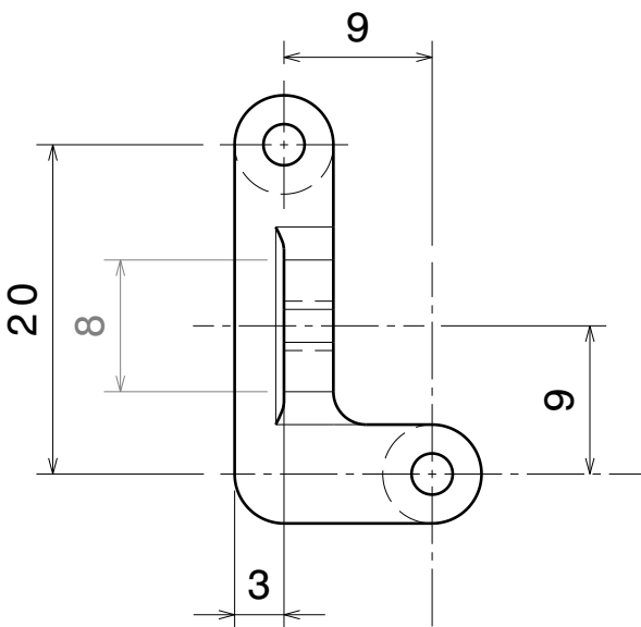
Top view Scale: 2:1
