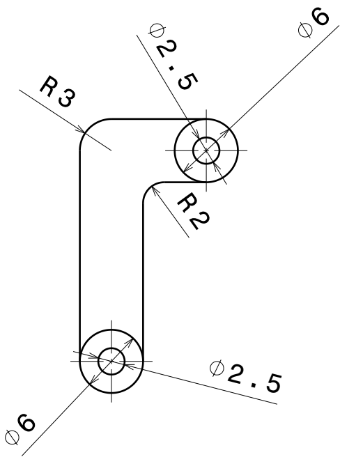
Bottom view Scale: 2:1
