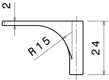
Right view Scale: 1:1
