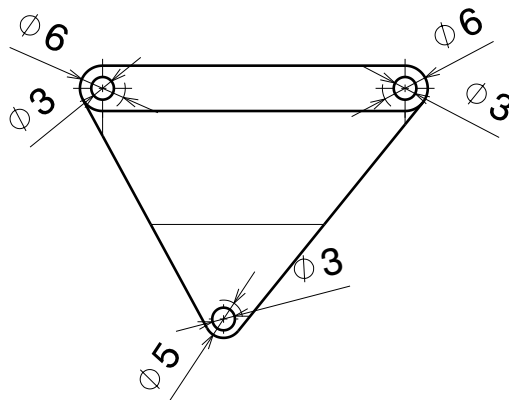
Top view Scale: 1:1
