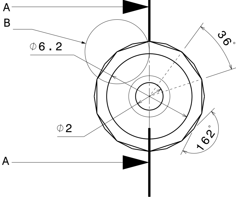
Vue de face Echelle : 6:1
