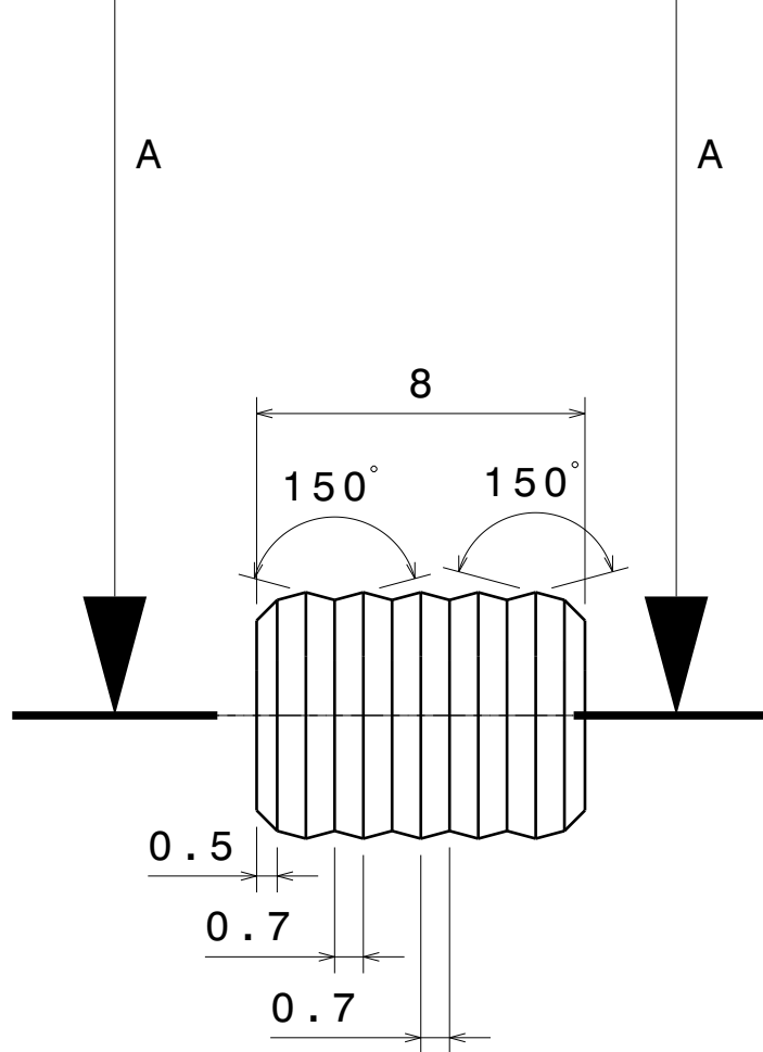
Vue de gauche Echelle : 5:1
