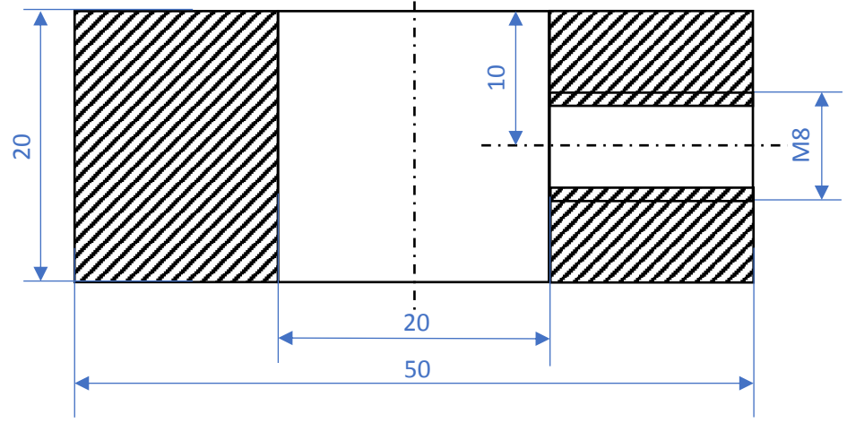
COUPE A-A
