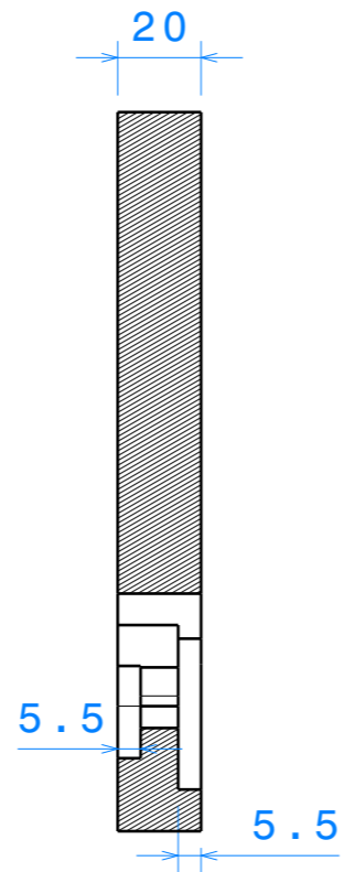
Section view A-A Scale: 1:2
