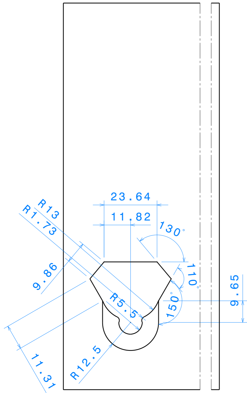
Back view Scale: 1:1
