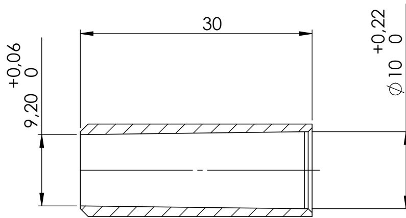
COUPE A-A
