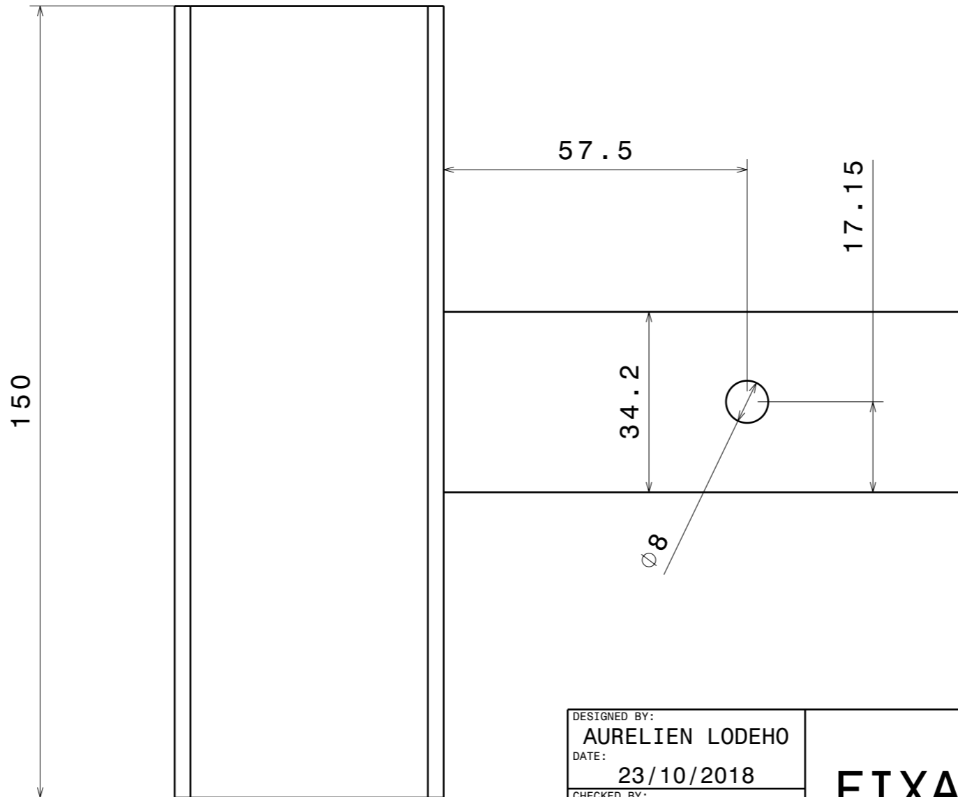
Vue de face Echelle : 1:1
