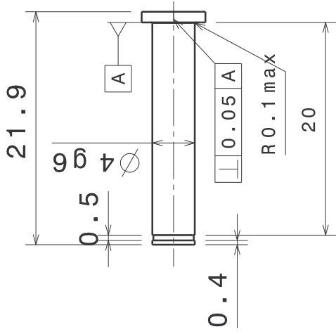
Vue de face Echelle : 2:1
