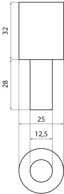
REF AXE-25 Acier trempé 2 Unités
