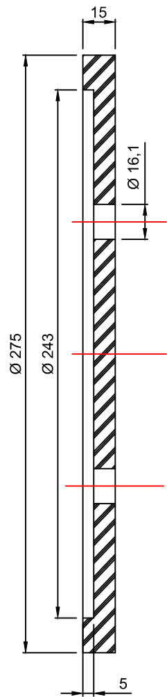
Coupe AA
