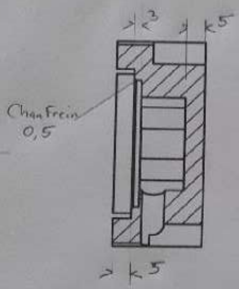
A-A (1:1)
