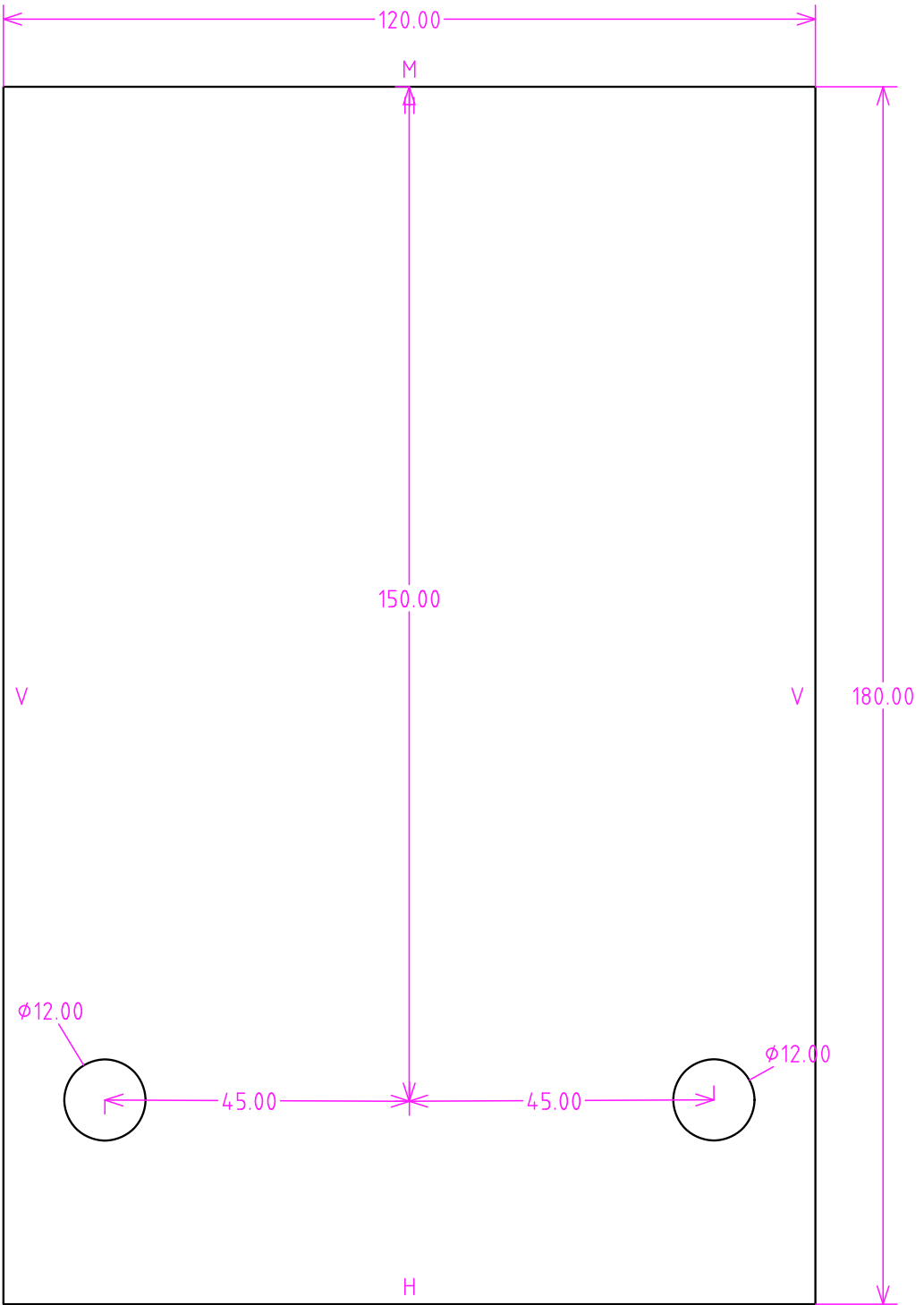
Plaque type 2 - Acier - Epaisseur 5 mm
