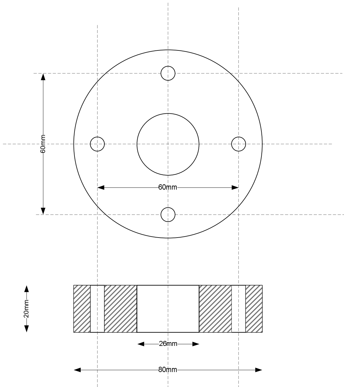
Bride plate acier ordinaire Ø80mm, 1 trou central Ø 26mm 4 trous Ø 6mm Aucun traitement Tolérances de perçage: -0+0,1mm
