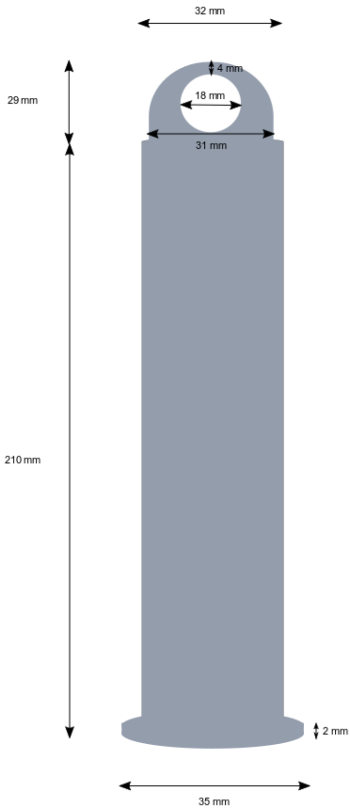
Vue Profil
