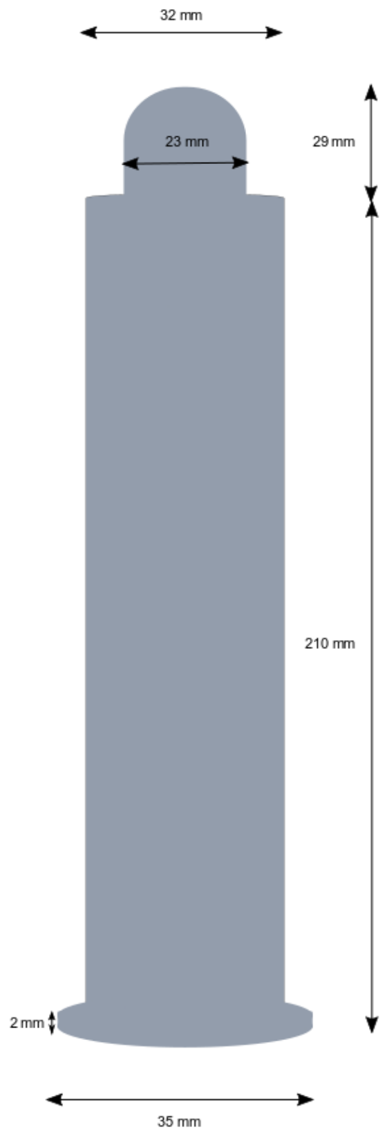
Vue face
