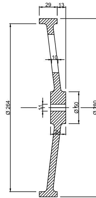
Coupe AA
